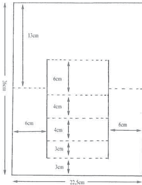
Schneide- und Falzskizze
